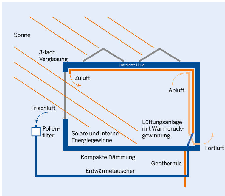
Funktionsweise einer Sporthalle, gebaut im Passivhaus-Standard.
