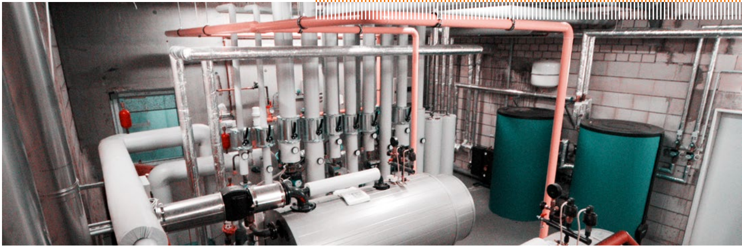
Heizungskeller: Der Heizkessel sollte auf dem aktuellen Stand der Technik sein. Aber das Augenmerk richtet sich auch auf unnötige Energiebrücken.
